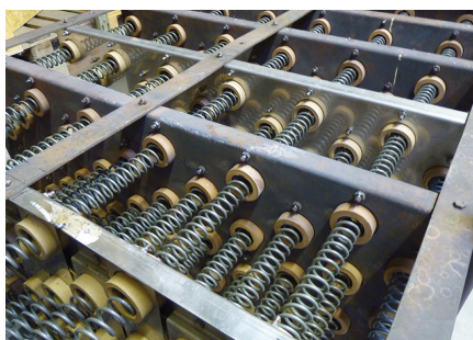
Reparatur Luftheizregister
